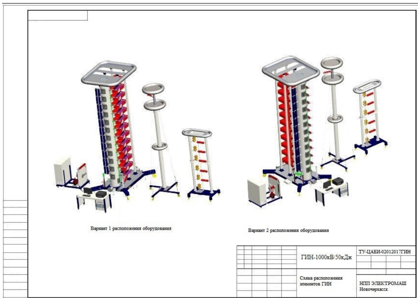
Схема расположения элементов ГИН
