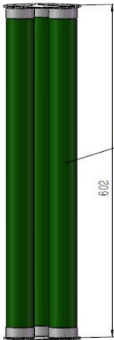
Резистор высоковольтный РВ-100-3-1.ЦАЕИ 52×598мм
