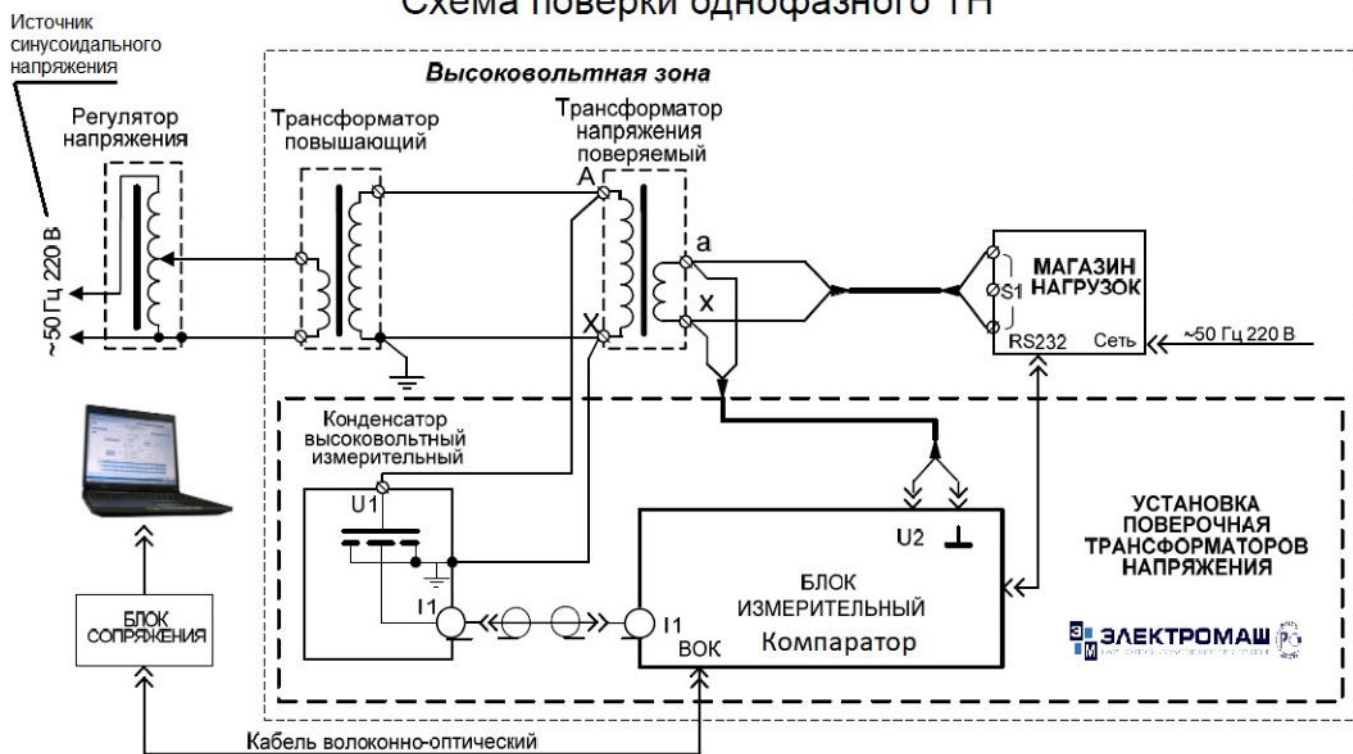
Схема проверки однофазного ТН
