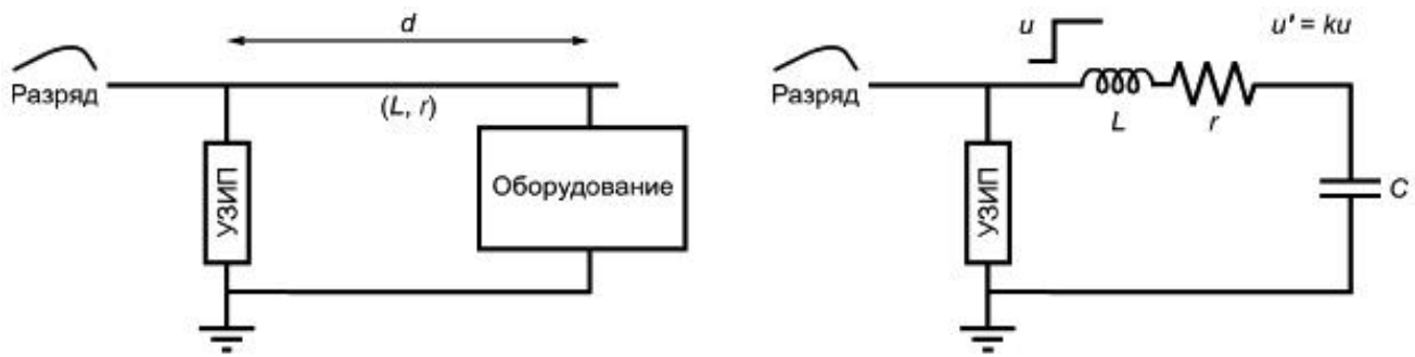
Рисунок К.8 - Физическая и электрическая схемы системы, в которой защищаемое оборудование отделено от УЗИП, осуществляющего защиту
