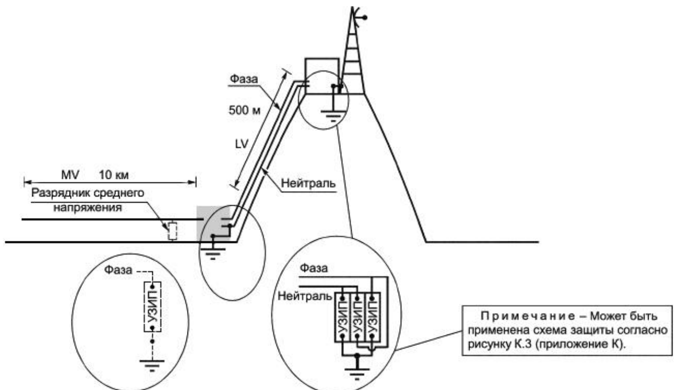
Рисунок Г.4 - Установка с системой молниезащиты
