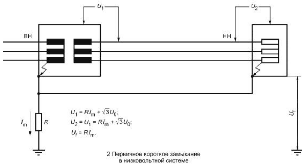
Рисунок Е.10 - Система IT, пример е2
