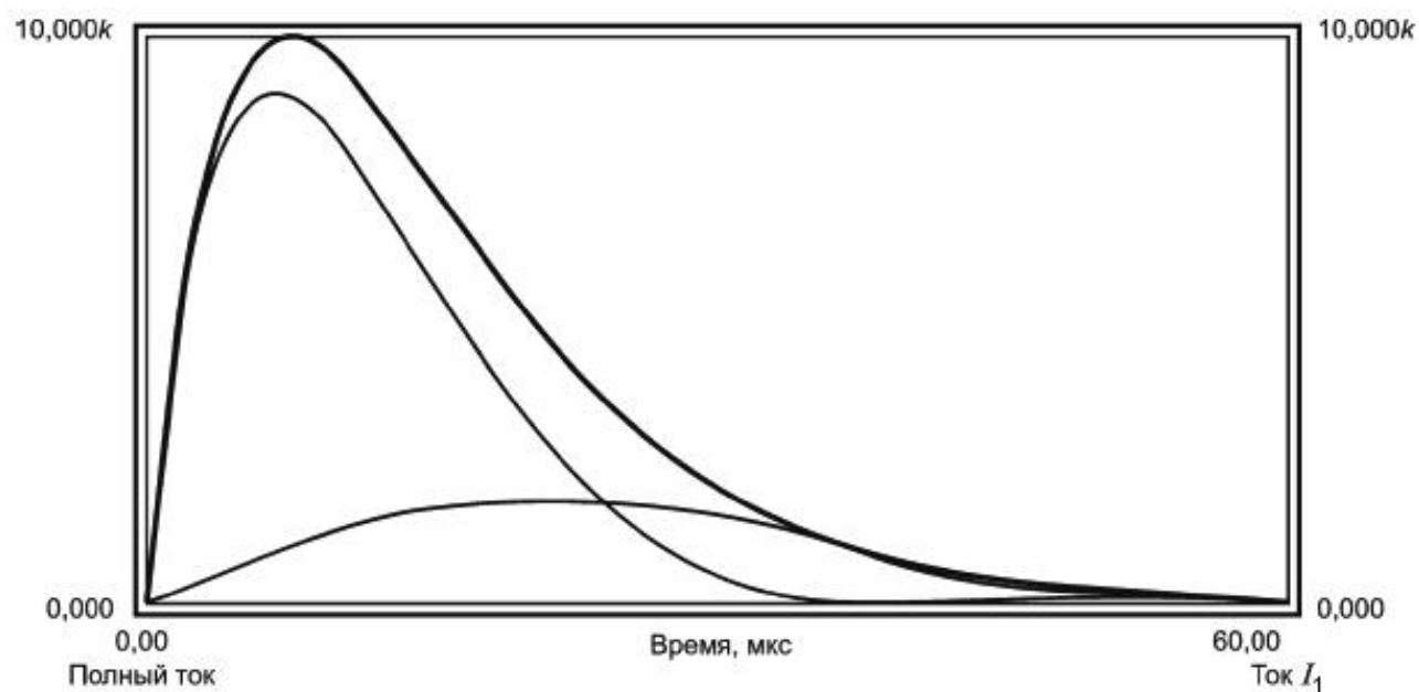
Рисунок К.12 - Координация двух цинкооксидных варисторов
