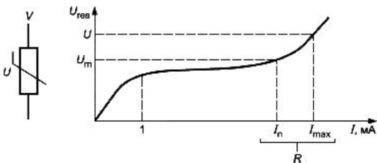
Рисунок 7 - Типичная кривая U(\text{res})/I варисторов на основе окиси цинка
