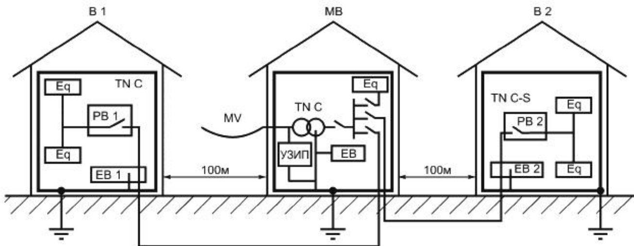
Рисунок G.2 - Пример распределительных сетей промышленного объекта
