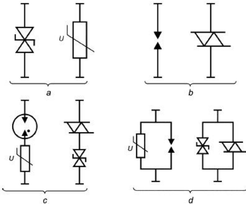
Рисунок 5 - Примеры элементов и комбинаций элементов
