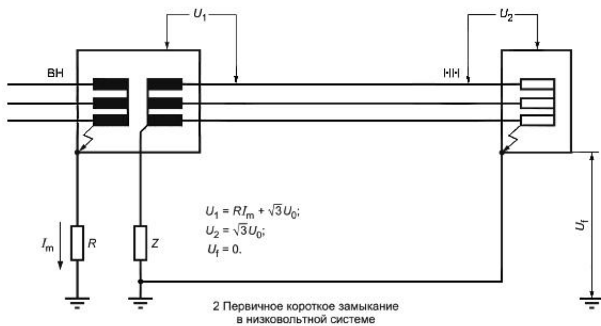
Рисунок Е.8 - Система IT, пример d
