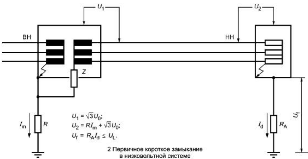
Рисунок Е.5 - Система IT, пример б
