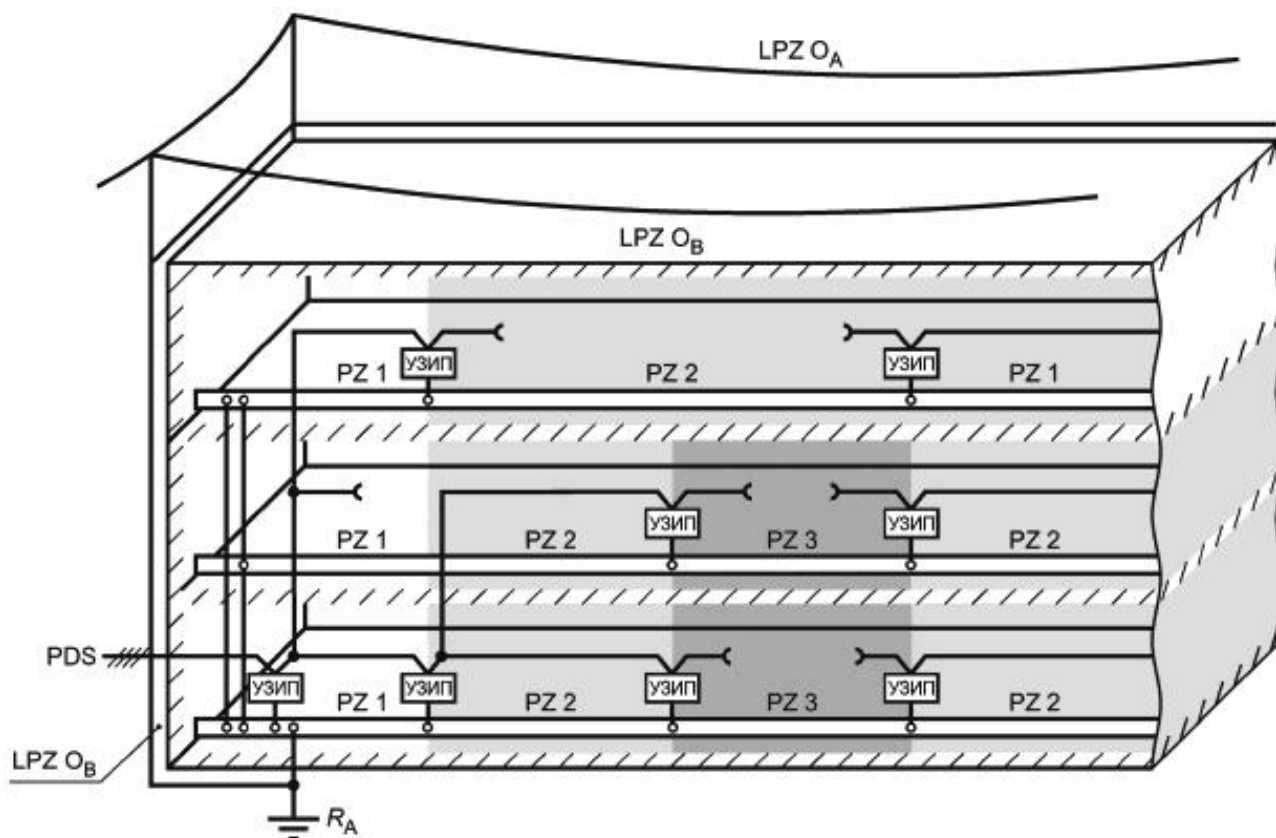
Рисунок К.11 - Деление здания на зоны защиты
