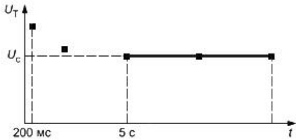
Рисунок J.1 - Типичная кривая U_T для УЗИП
