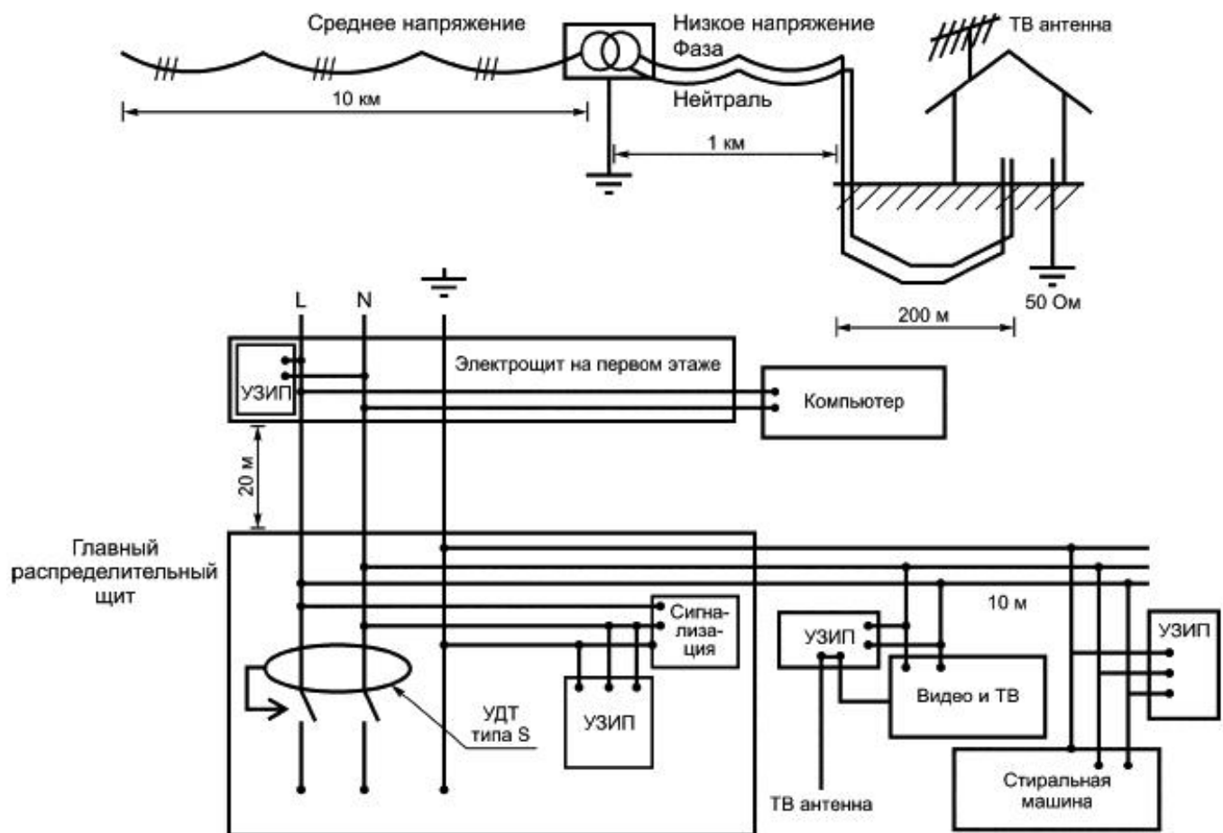
Рисунок G.1 - Бытовая электроустановка
