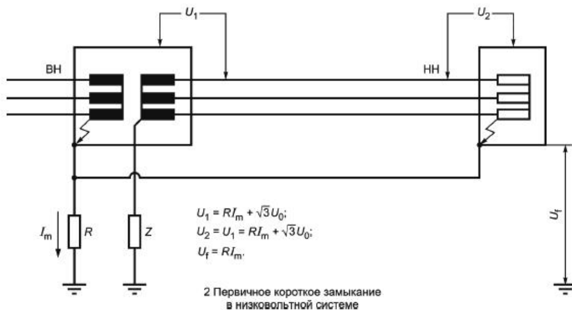
Рисунок Е.9 - Система IT, пример е1
