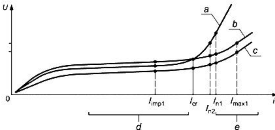
Рисунок F.2 - Два цинкооксидных варистора с разными номинальными разрядными токами
