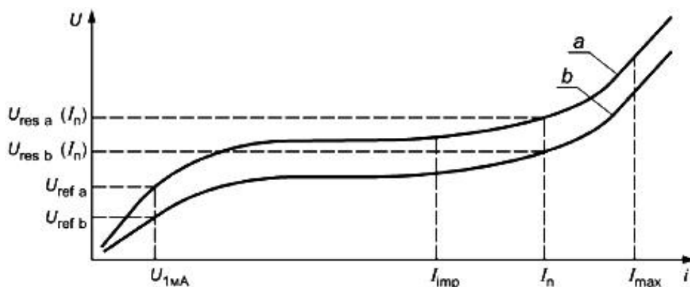
Рисунок Ф.1 - Два цинкооксидных варистора с одинаковым номинальным разрядным током
