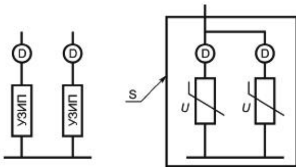
Рисунок J.3 - Применение параллельных УЗИП
