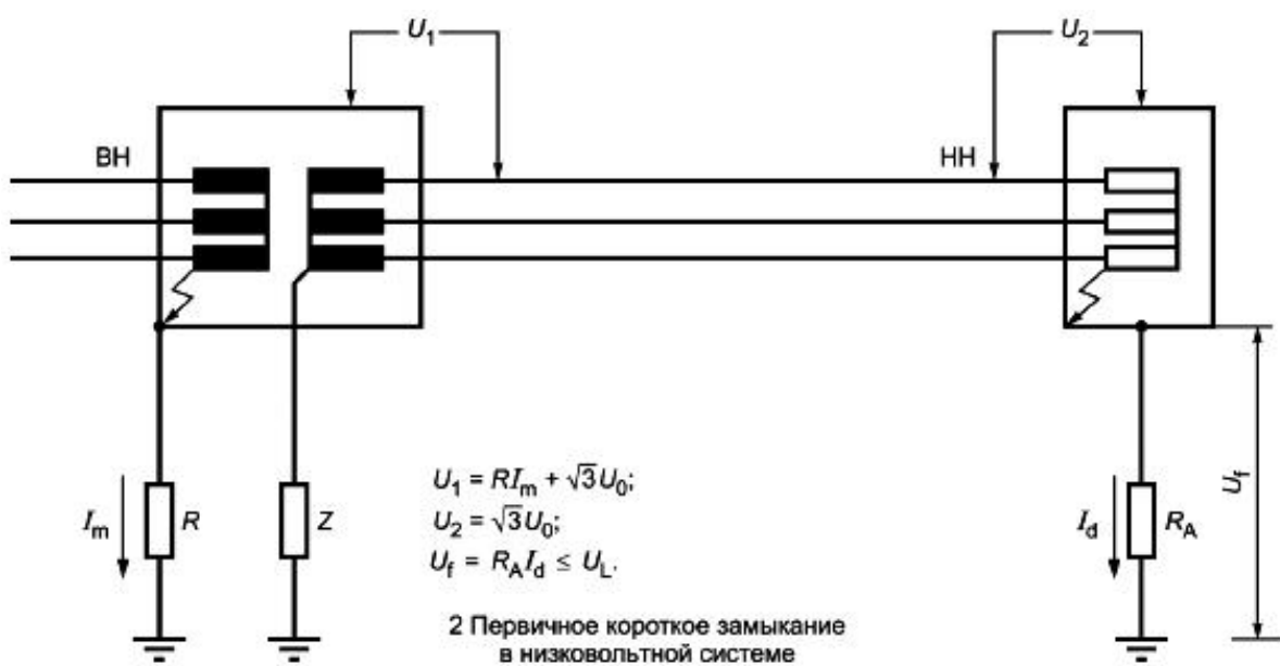
Рисунок Е.6 - Система IT, пример с1
