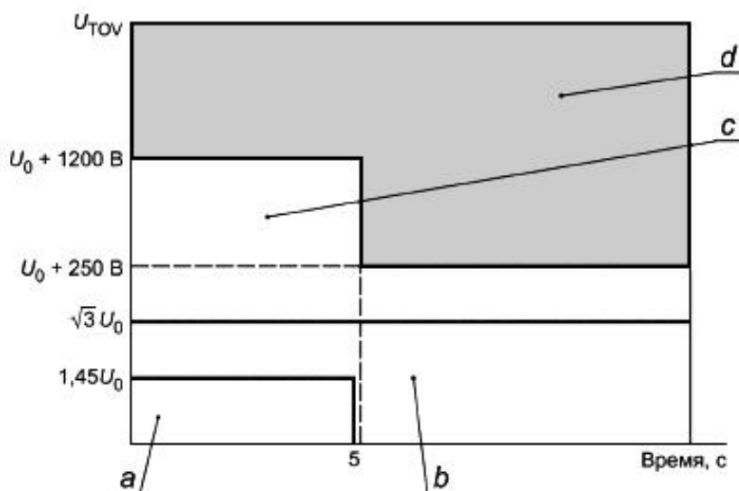
Рисунок 4 - Максимальные значения U(TOV) согласно МЭК 60634-4-44
