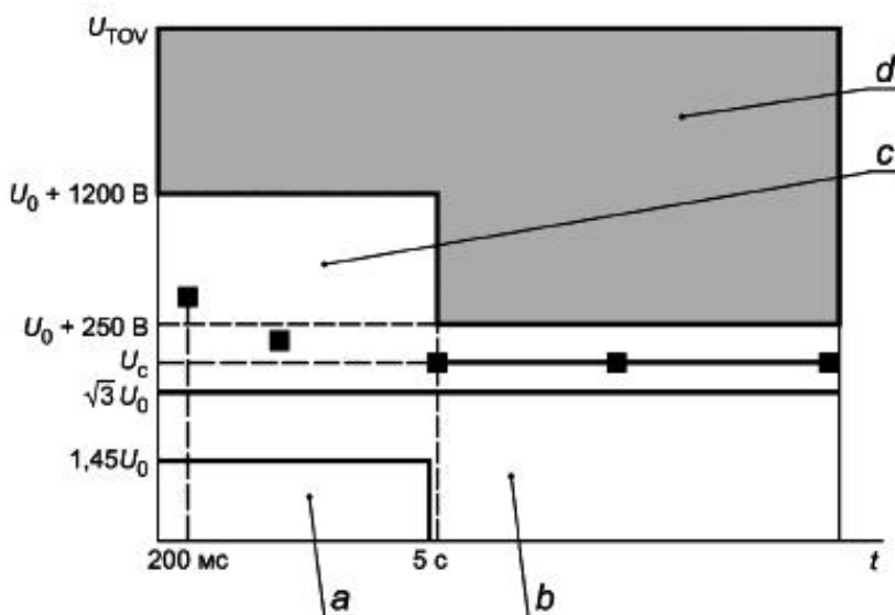
Рисунок 13 - Соотношение U(T) и U(TOV)
