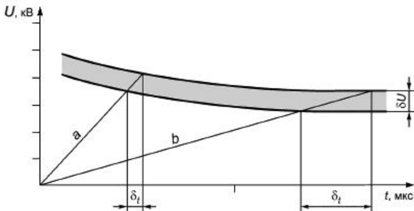
Рисунок 8 - Типичная кривая разрядника
