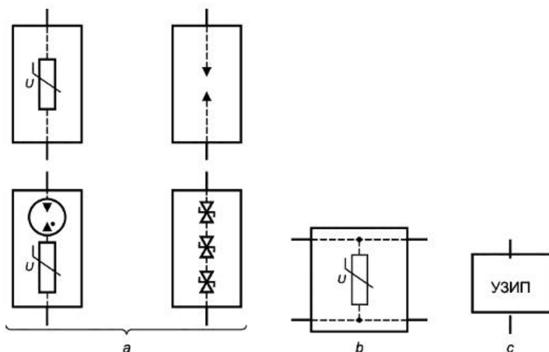
Рисунок 1 - Примеры обозначений однофазных УЗИП
