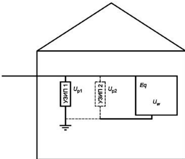
Рисунок 11 - Необходимость дополнительной защиты
