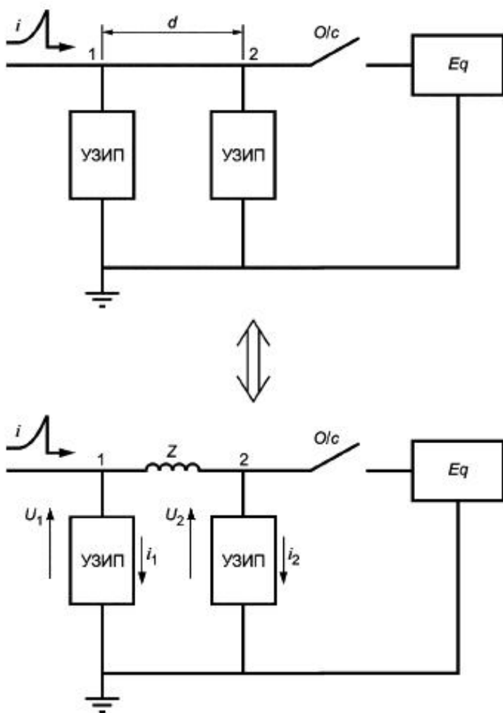
Рисунок 14 - Типичный пример применения двух УЗИП - электрическая схема
