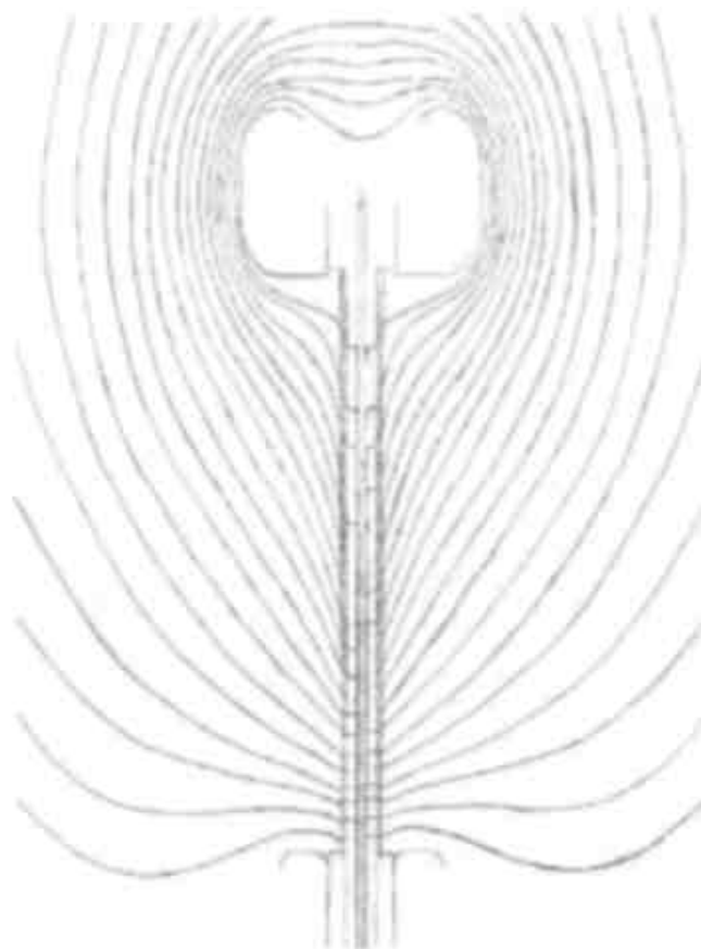
Стандартное распределение поля в концевом устройстве
