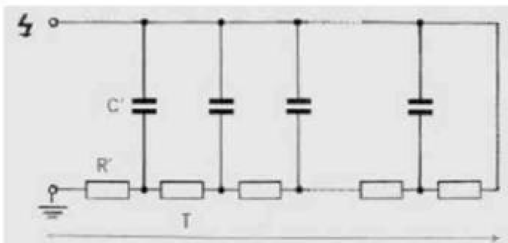
Эквивалентная схема цепи испытаниях концевых устройств
