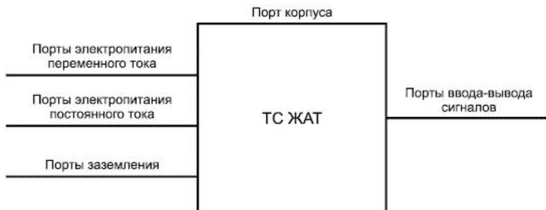
Рисунок 1 - Примеры портов ТС ЖАТ
