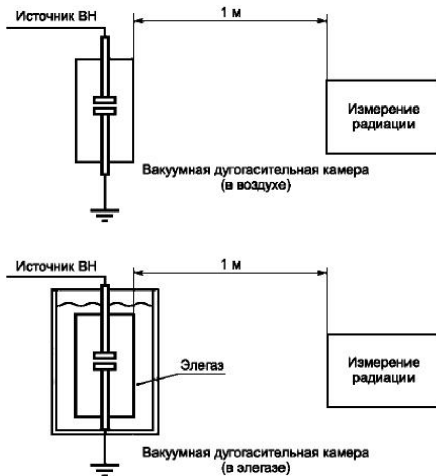
Рисунок 2 - Место монтажа дозиметра
