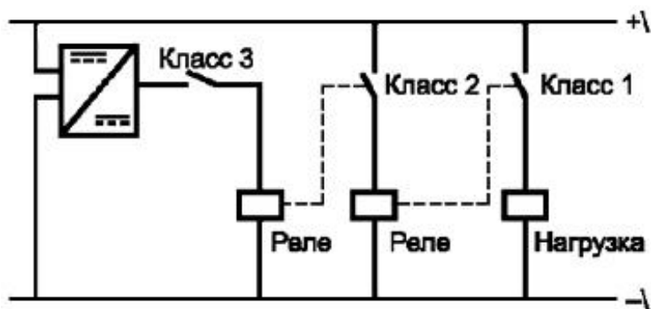
Рисунок 1 - Примеры классов контактов
