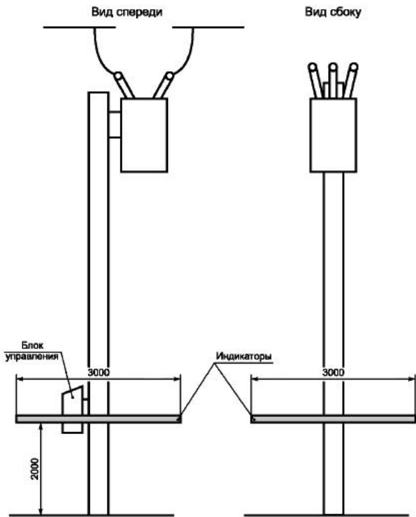
Рисунок А.7 - Испытательная установка для КРУ, монтируемого на столбе
