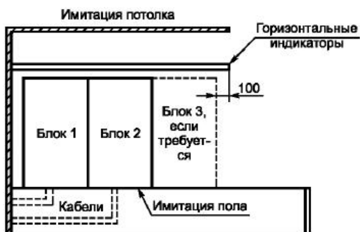
Вид спереди
