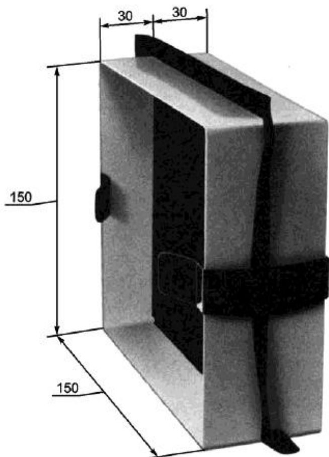
Рисунок А.1 - Монтажная рамка для вертикального индикатора
