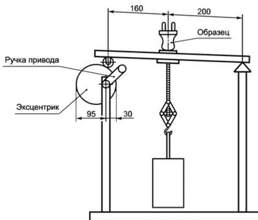
Рисунок 8 - Установка для испытания крепления шнура
