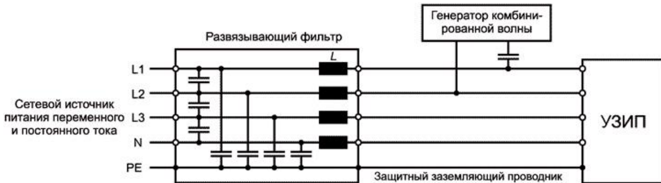
Рисунок 2 - Пример развязывающего фильтра для трехфазной сети
