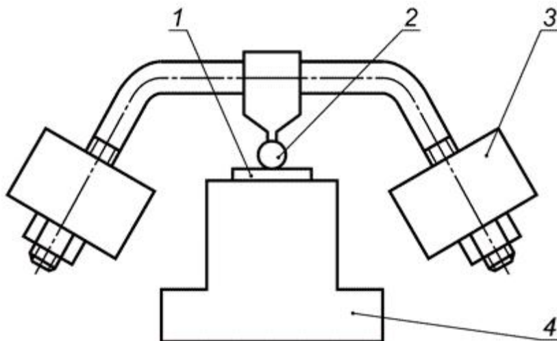
Рисунок 12а - Установка для испытания давлением шарика
