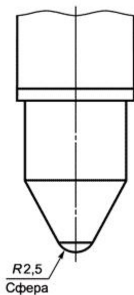
Рисунок 12б - Нагрузочный стержень для испытания давлением шарика
