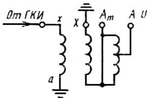
Испытание однофазного автотрансформатора
