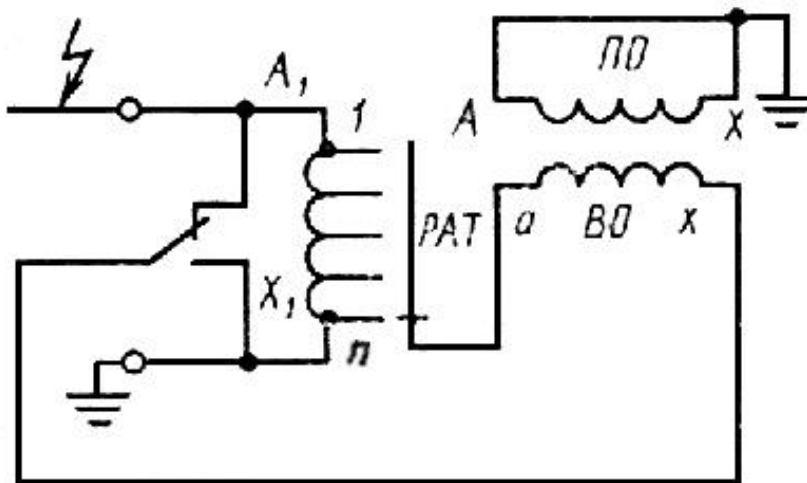
PAT - регулировочный трансформатор
