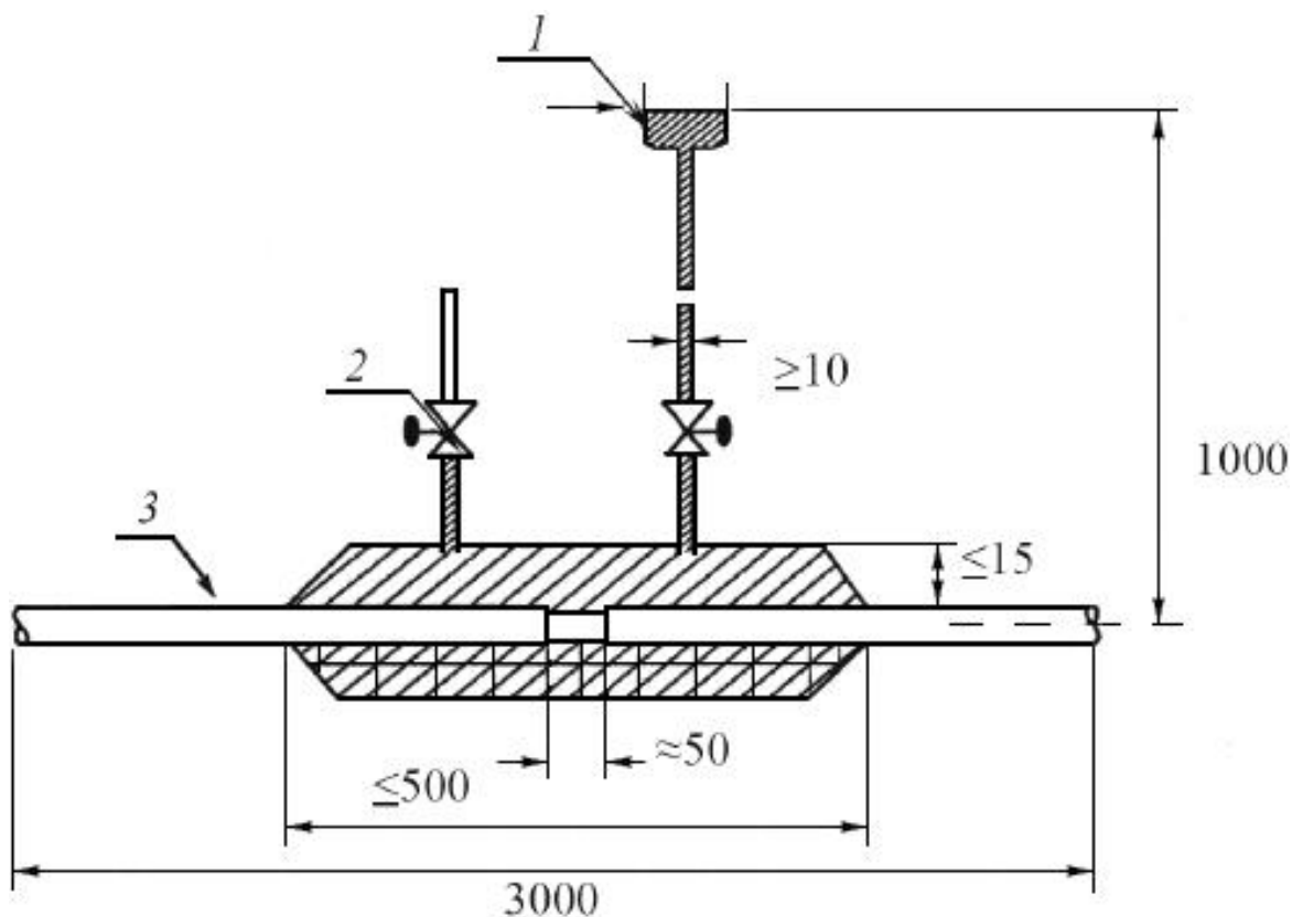
Рисунок 3 - Схема устройства для испытания на продольное распространение воды
