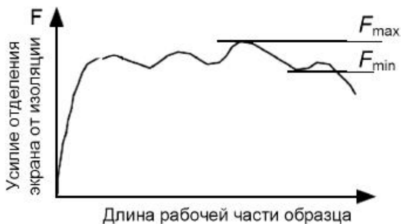
Рисунок 2 - Усилие отделения электропроводящего экрана от изоляции
