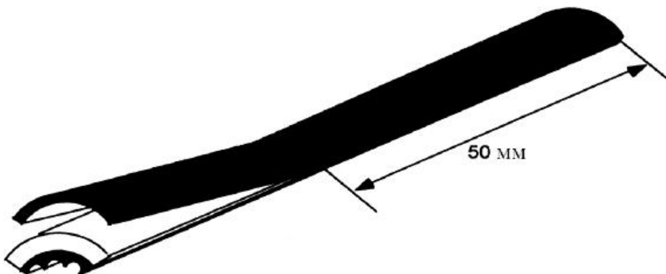
Рисунок 1 - Проверка отделяемости экструдированного электропроводящего экрана
